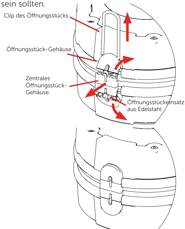
Diagramm für den Austausch von QuickFlight-Öffnungsstücken (Gurtband nicht abgebildet)
