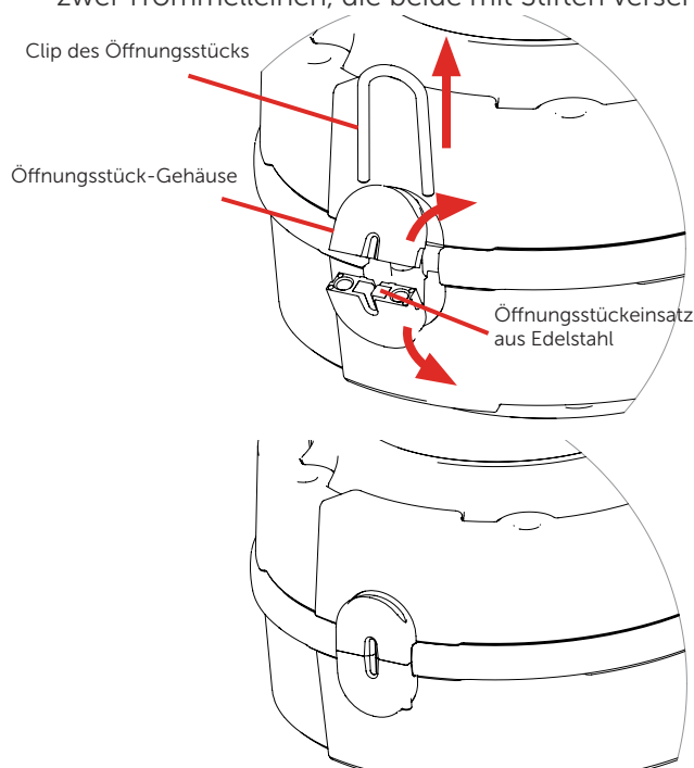
Diagramm für den Austausch von Ein-Leinen-Öffnungsstücken (Gurtband nicht abgebildet)
