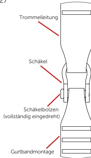
Gurtband-Schäkel-Verbindung
