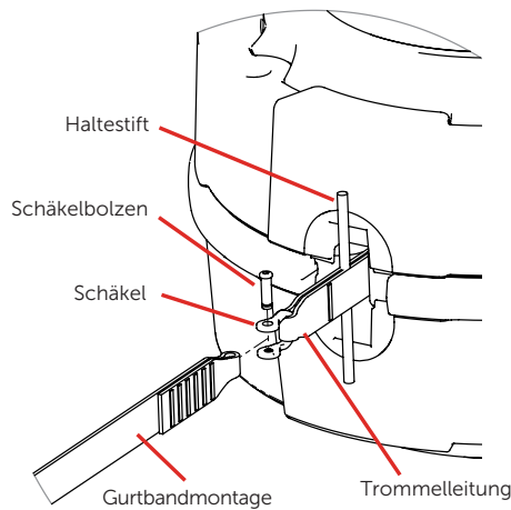
Einfache Trommelleine
